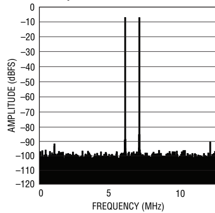
LTC2263-12: 8k Point 2-Tone FFT, f_{IN} = 68\text{MHz} , 69\text{MHz} , -1\text{dBFS} , 25\text{Mps}
