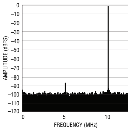
LTC2263-12: 8k Point FFT, f_{IN} = 140\text{MHz} , -1\text{dBFS} , 25\text{Mps}
