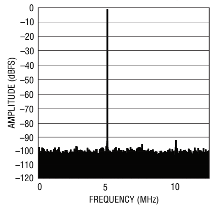
LTC2263-12: 8k Point FFT, f_{IN} = 70\text{MHz} , -1\text{dBFS} , 25\text{Mps}
