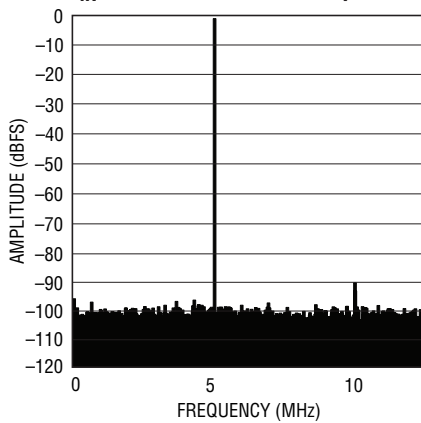
LTC2263-12: 8k Point FFT, f_{IN} = 5\text{MHz} , -1\text{dBFS} , 25\text{Mps}
